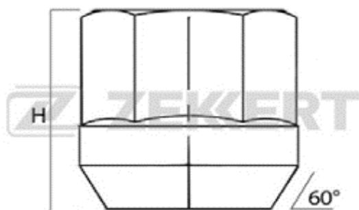
Closed lug nuts cone seat 17 hex / Гайки колесные закрытые, конус, ключ 17
