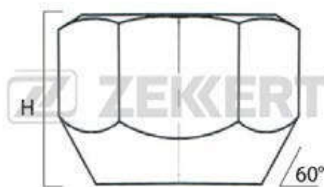
Open lug nuts cone seat 19 hex / Гайки колесные открытые, конус, ключ 19
