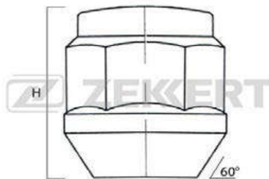
Closed lug nuts cone seat 19 hex / Гайки колесные закрытые, конус, ключ 19
